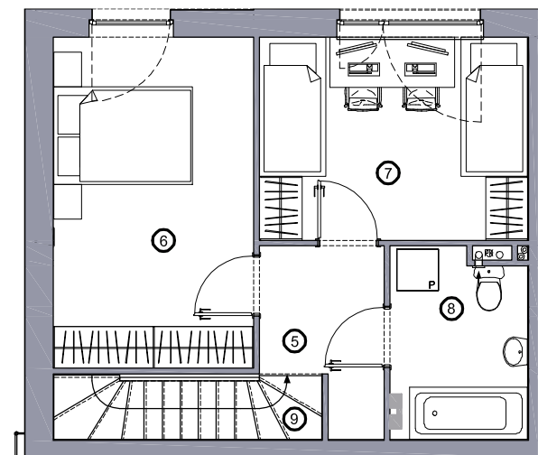
Rzut 1 piętra
